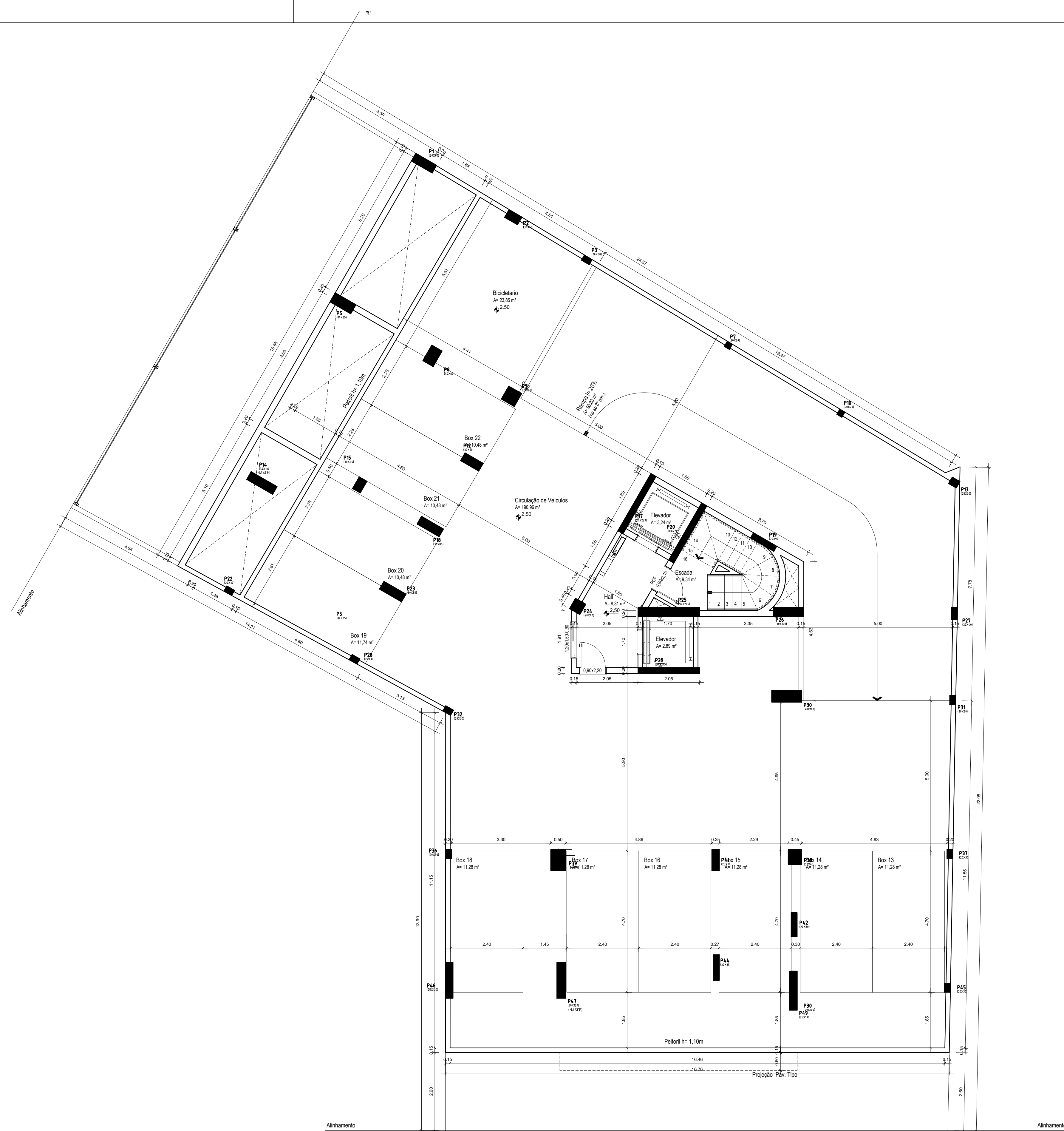
Planta Baixa 2º Pav (Boxes) Esc. 1/75
