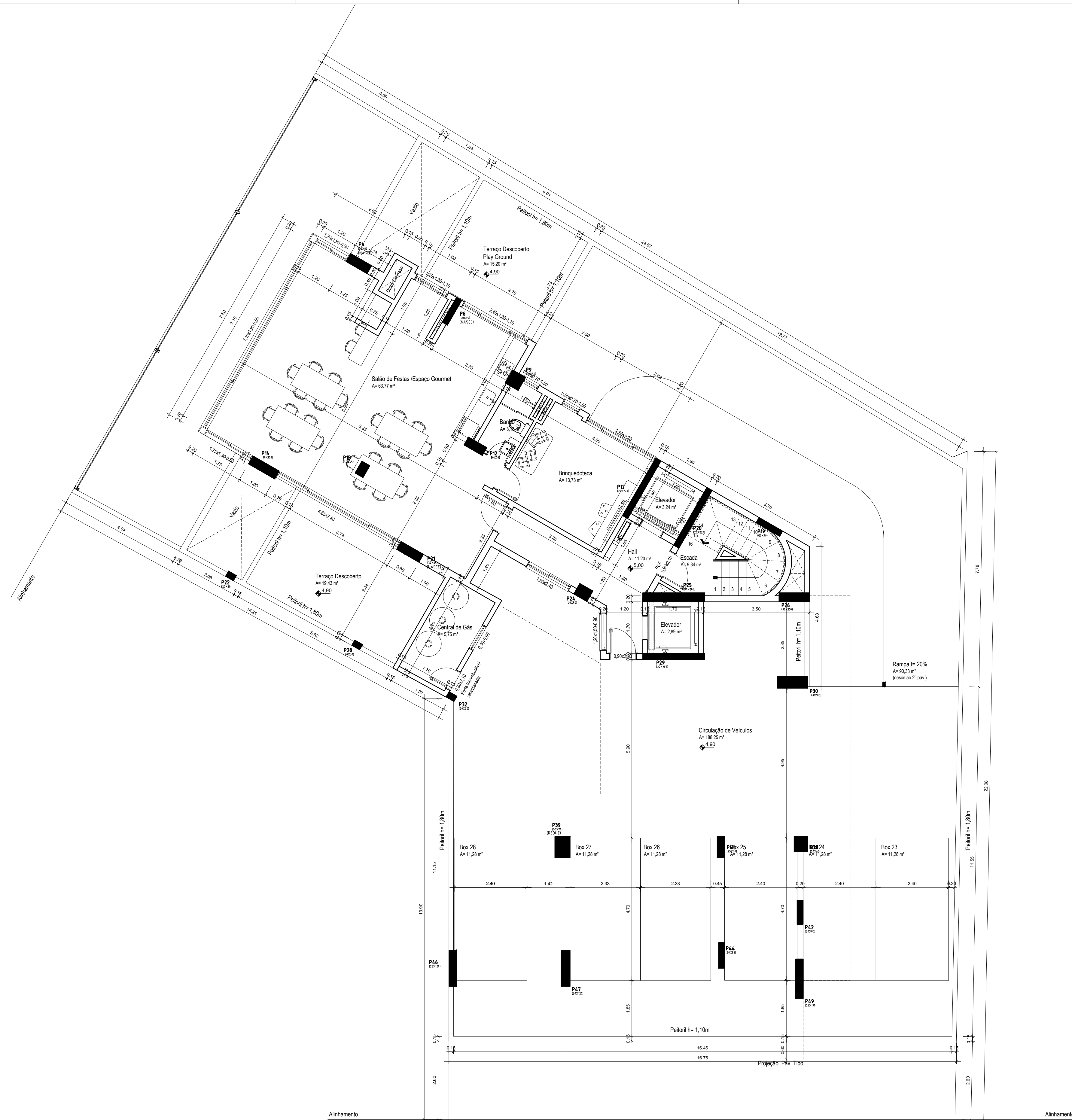
Planta Baixa 3º Pav. ( Áreas de uso comum ) Esc. 1/75
